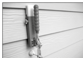
3. Montageklem voor CEDRAL
